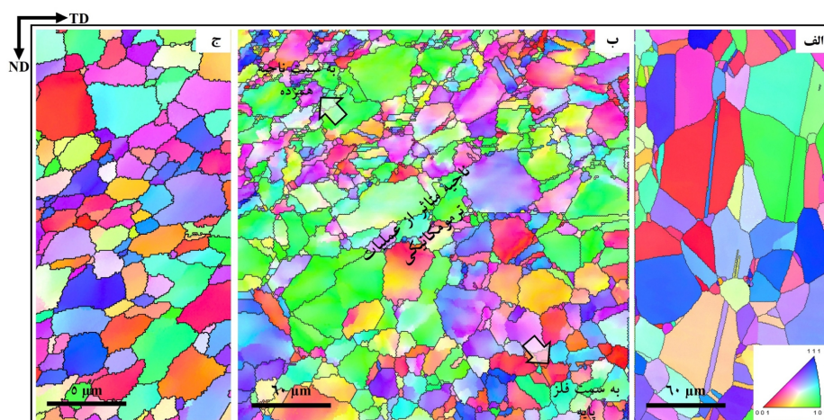
شکل 2- نقشه های جهت گیری از فلز پایه (الف) فلز پایه، (ب) سمت پیشرونده ناحیه همزده، و (ج) ناحیه همزده
