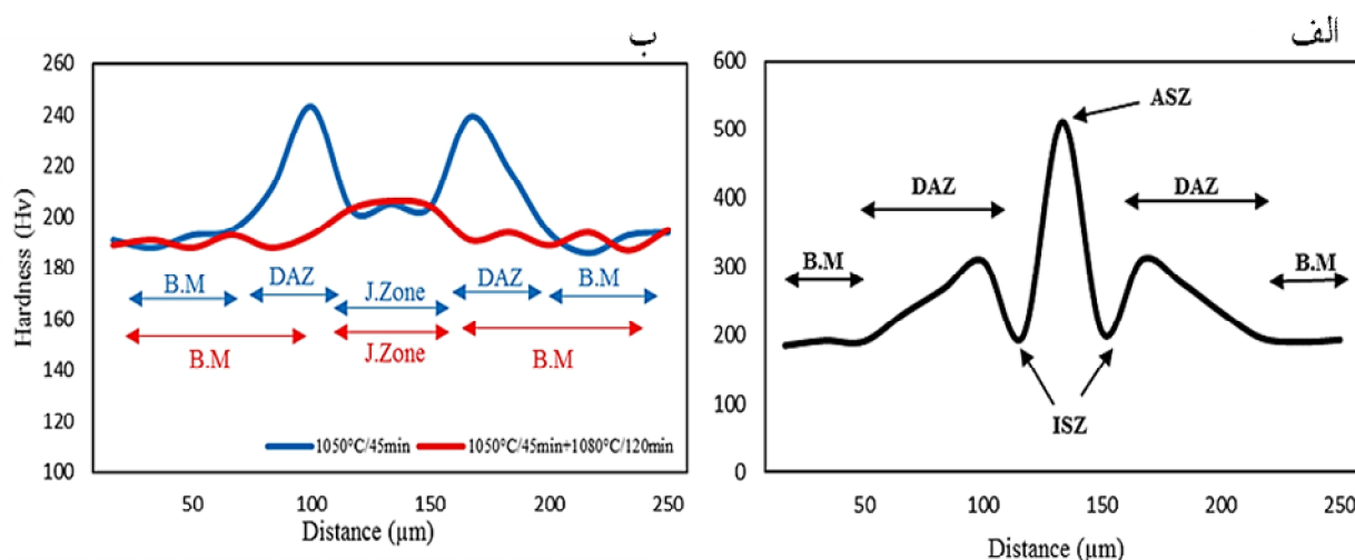
شکل 8. پروفیل سختی اتصال مشابه اینکونل 600 (الف) دمای 1050 و زمان 5 دقیقه (ب) اتصالات همگن سازی شده.
