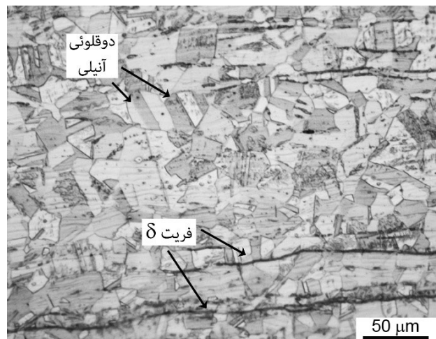
شکل 1- تصویر میکروسکوپی نوری از ریزساختار فلز پایه فولاد آستیتی 304 L (فريت d و دوقلوئی های آئیلی با پیکان مشخص شده اند).
